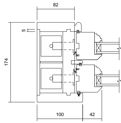
03 Jamb Detail 1 : 5
