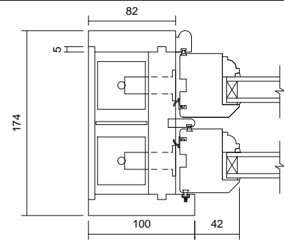
03 Jamb Detail 1 : 5
