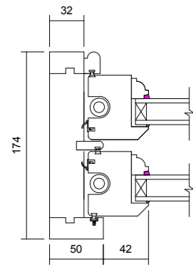
03 Jamb Detail 1 : 5
