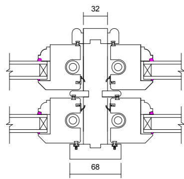
04 Mullion Detail 1 : 5
