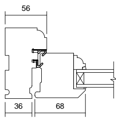
03 Jamb Detail 1 : 5
