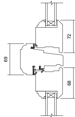
06 Transom Detail 1 : 5
