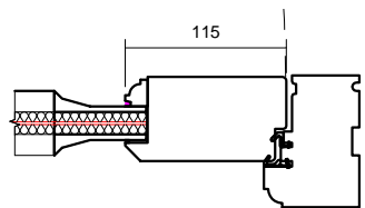
05 RH Jamb Detail 1 : 6
