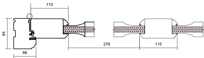
03 LH Jamb Detail 1 : 6
