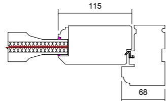
05 RH Jamb Detail 1 : 6
