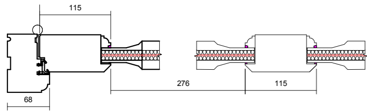
03 LH Jamb Detail 1 : 6
