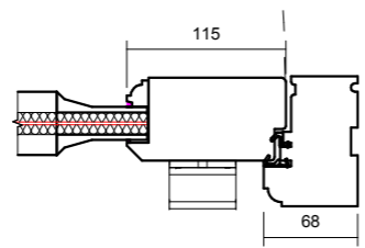
05 RH Jamb Detail 1 : 6
