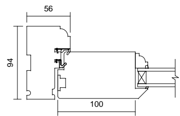
03 Jamb Detail 1 : 5
