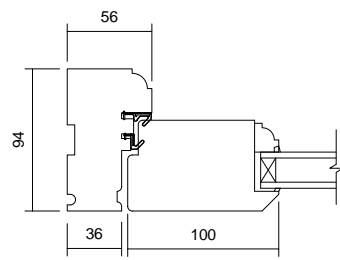
03 Jamb Detail 1 : 5
