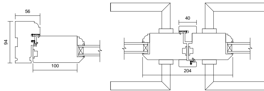
03 Jamb Detail 1 : 5
