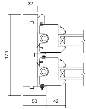
03 Jamb Detail 1 : 5
