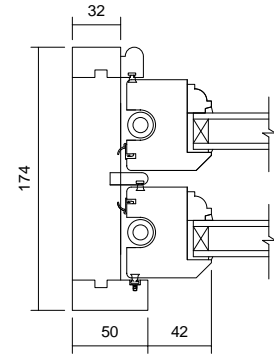
03 Jamb Detail 1 : 5
