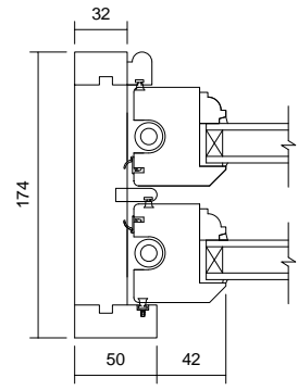
03 Jamb Detail 1 : 5
