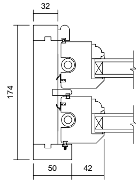
03 Jamb Detail 1 : 5
