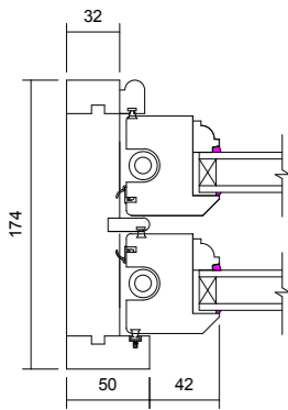
03 Jamb Detail 1 : 5
