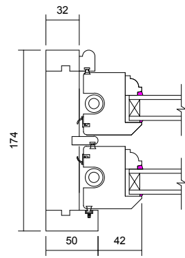
03 Jamb Detail 1 : 5
